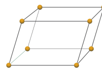
monoclinic
